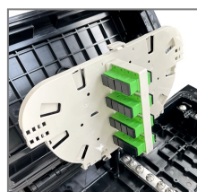
• Có thể gắn được Mini Naked Splitter • Gắn 16 adapters SC
